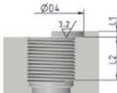
Setting DIN 3852-1
