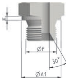
M DINBS Form A DIN 3852-1
