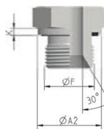
M DINE Form E DIN 3852-11
