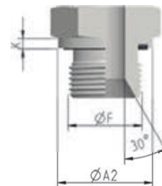
M DINE Form E DIN 3852-11
